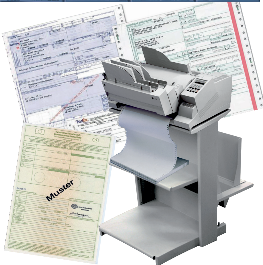
PP 405 mit Standfuß und 3 ASF Kassetten.
